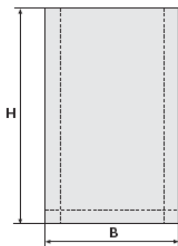
Figur 2 Pinchbotten med invikta sidor alt rak botten utan invikta sidor. I tabellerna anges måtten på produkter med invikta sidor som B/b \times H . Produkter utan invikta sidor anges som B \times H .
